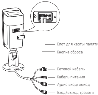
Рисунок 1. Описание цилиндрической камеры
