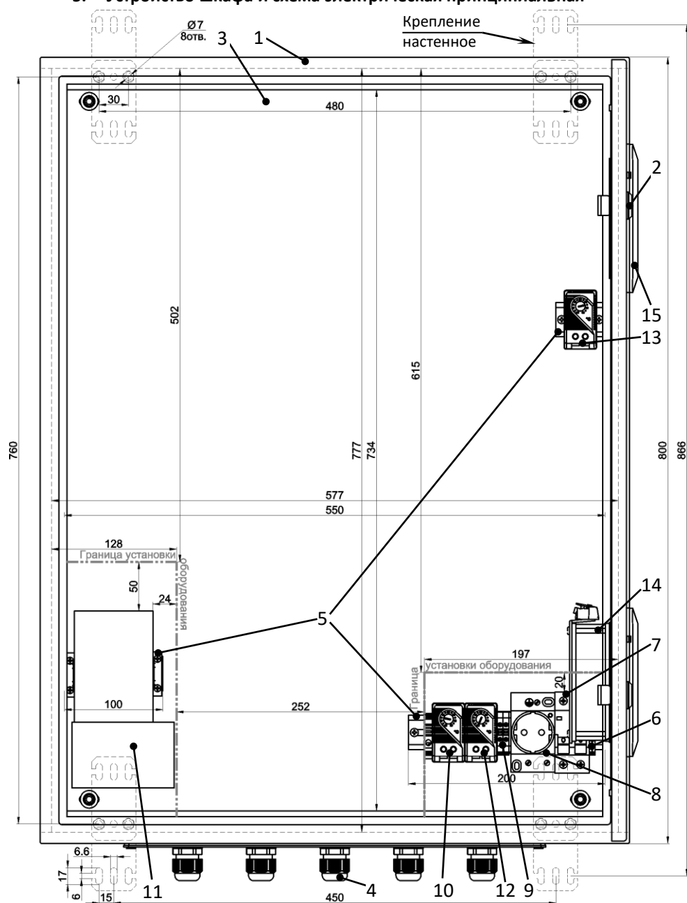
Рисунок 1 – Устройство шкафа
