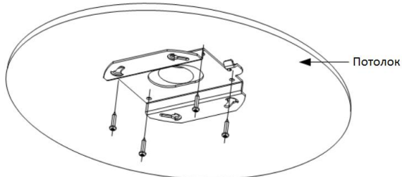
Рисунок 1-26 Установка потолочного крепления
