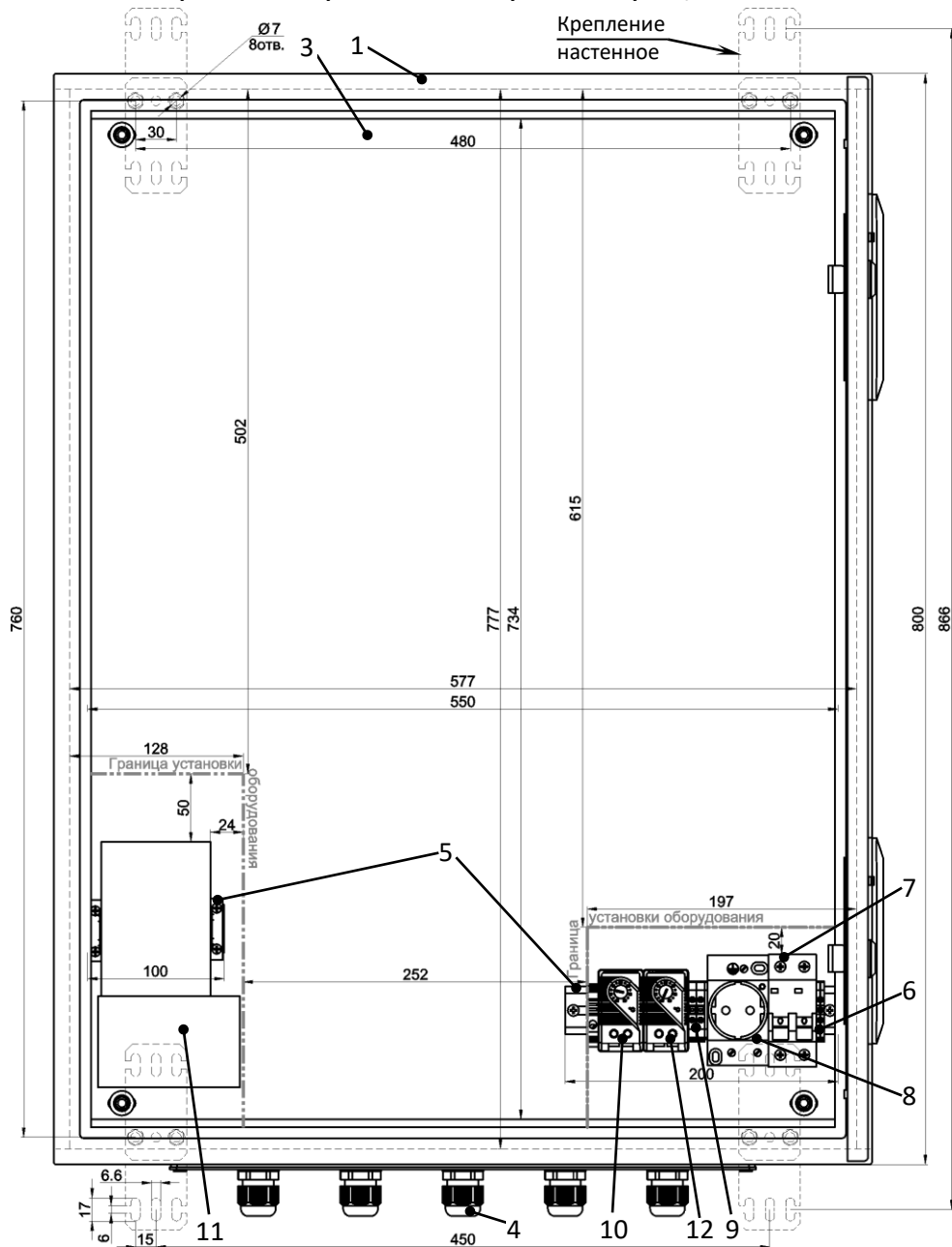
Рисунок 1 – Устройство шкафа
