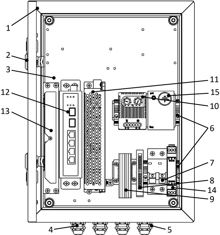
Рисунок 1 – Устройство шкафа
