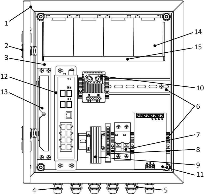
Рисунок 1 – Устройство шкафа
