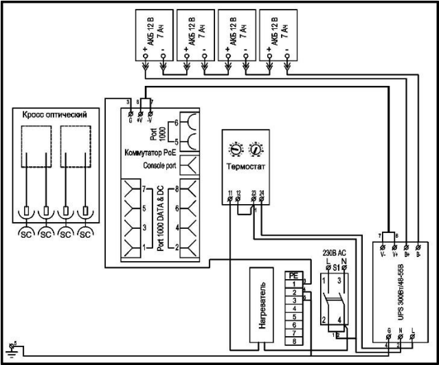
Рисунок 2 – Схема электрическая принципиальная
