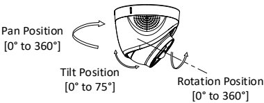
Рисунок 1-14 3-х осевая регулировка
