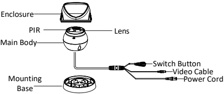
Рисунок 1-2 Обзор камеры II типа
