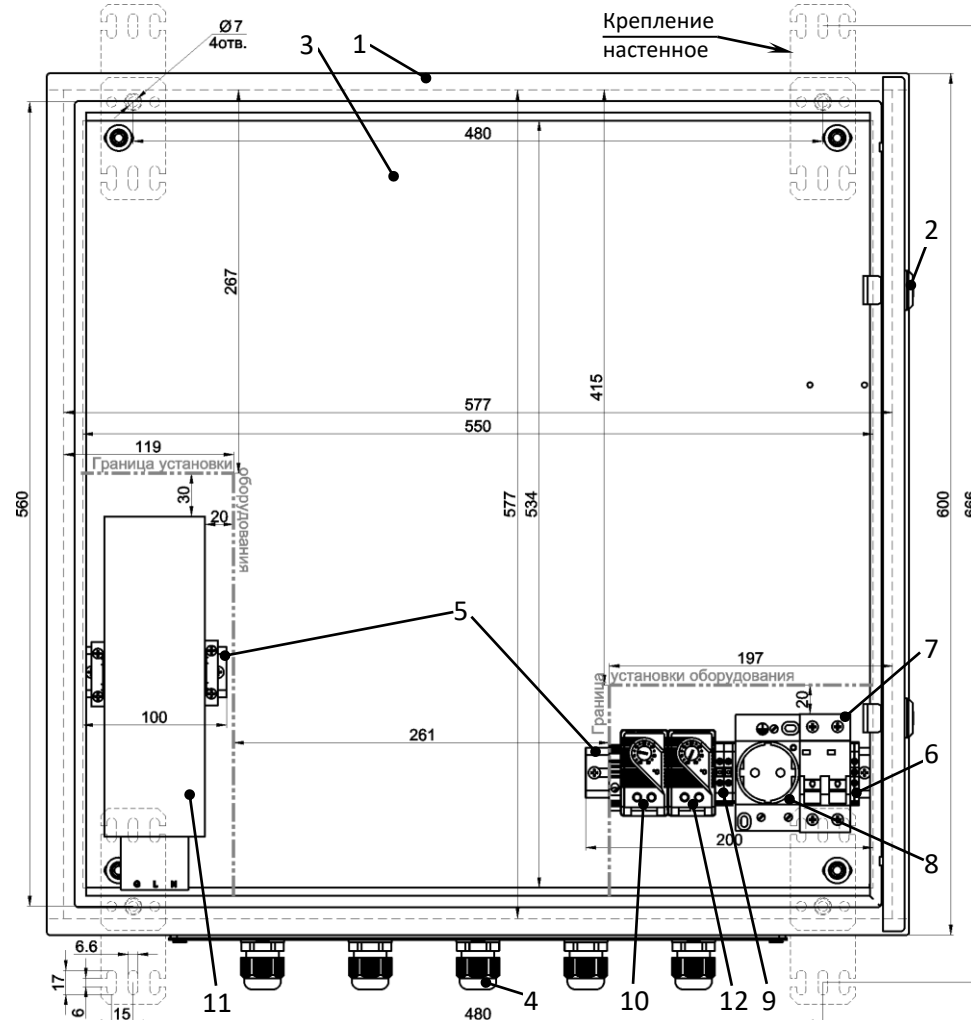
Рисунок 1 – Устройство шкафа
