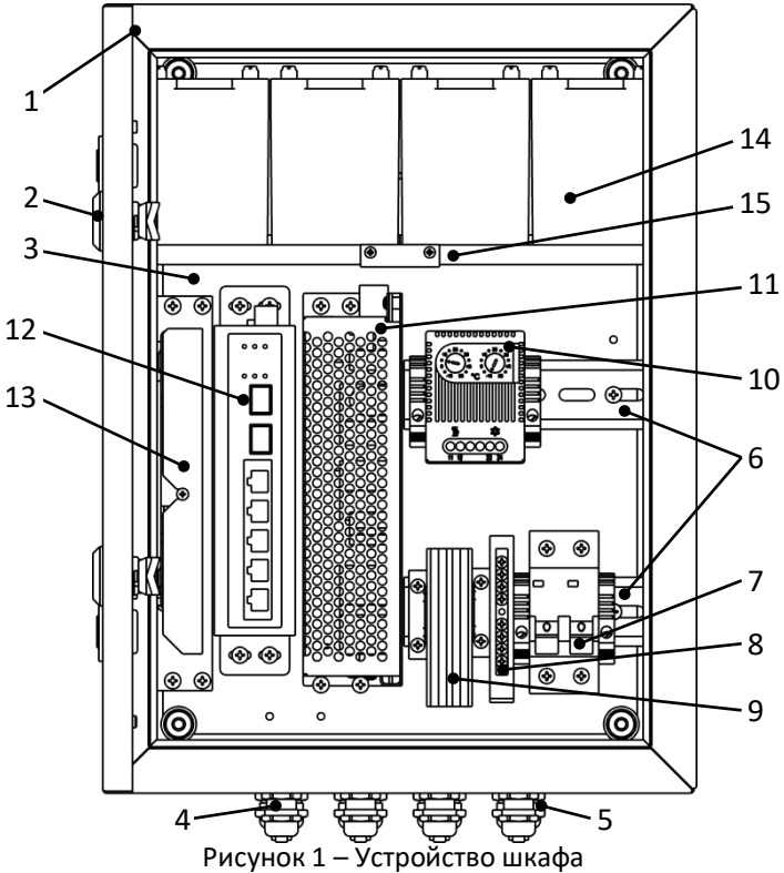
Рисунок 1 – Устройство шкафа
