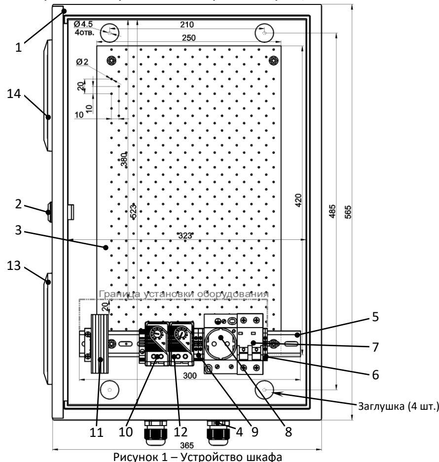
Рисунок 1 – Устройство шкафа
