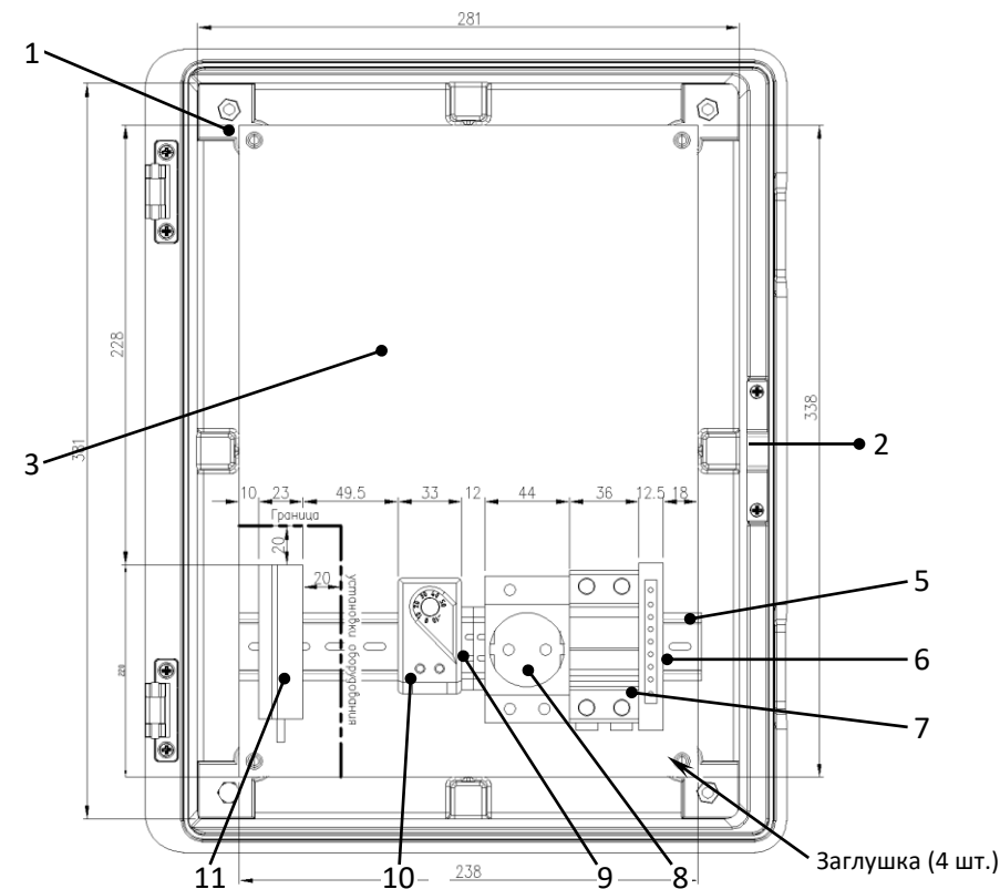
Рисунок 1 – Устройство шкафа
