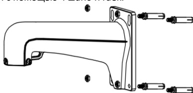
Рисунок 1-16 Установка кронштейна
