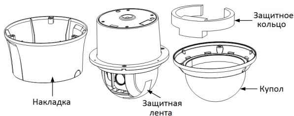
Рисунок 1-25 Демонтаж камеры
