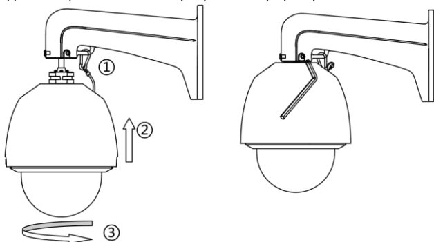
Рисунок 1-17 Установка скоростной поворотной камеры
