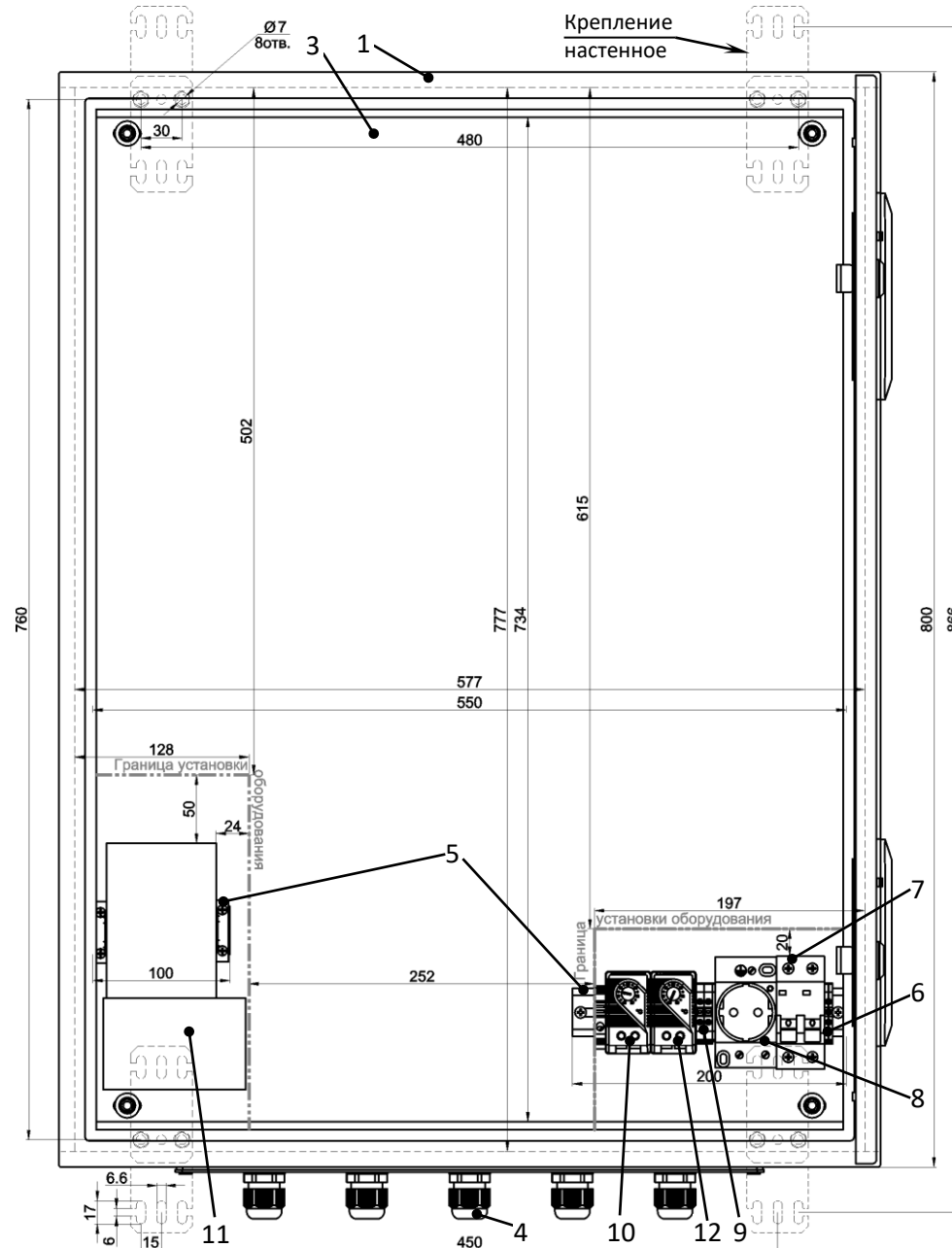
Рисунок 1 – Устройство шкафа
