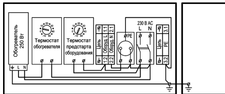
Рисунок 2 – Схема электрическая принципиальная
