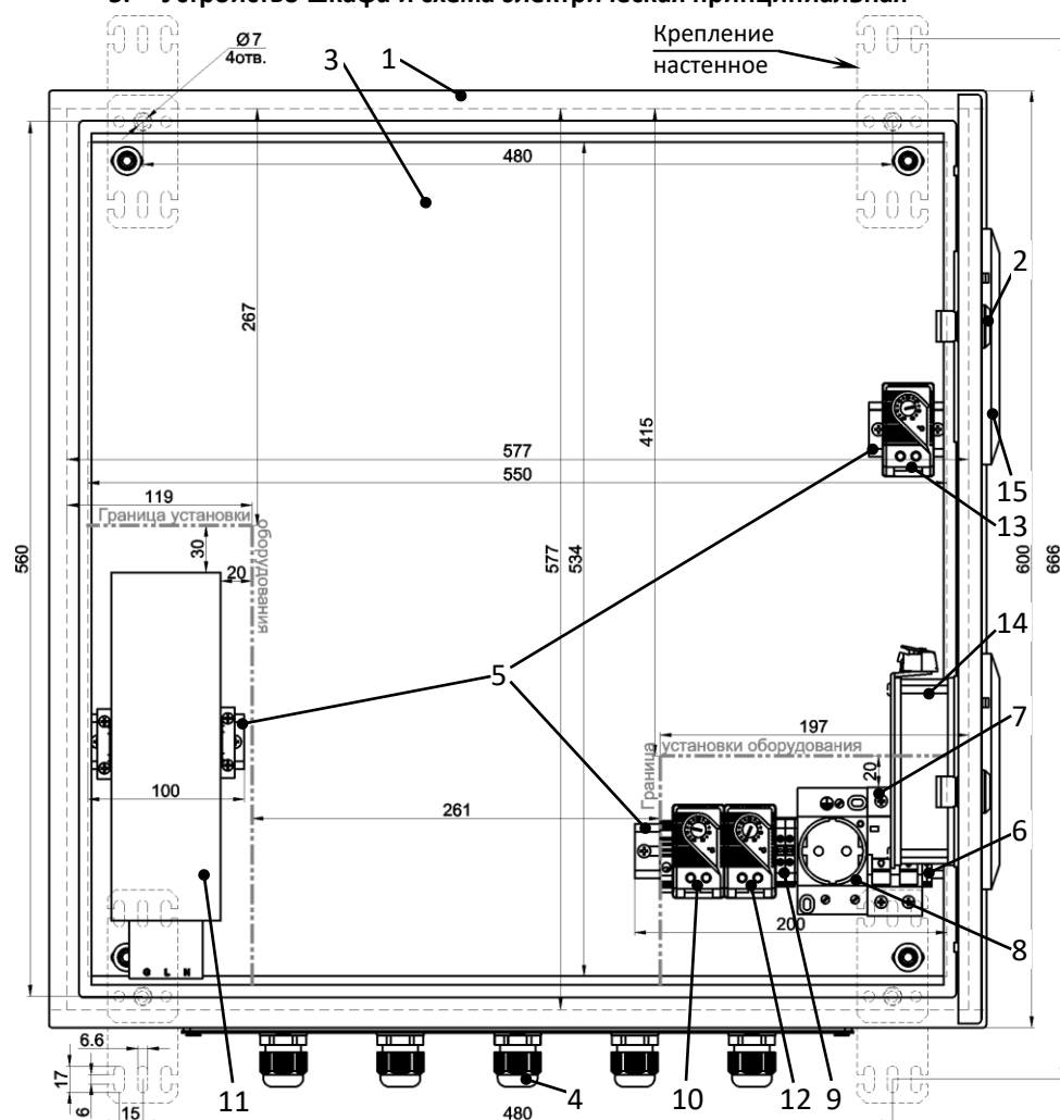
Рисунок 1 – Устройство шкафа
