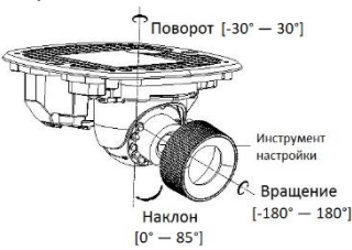
Рисунок 1-25 Настройка угла наблюдения камеры
