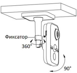
Рисунок 1-27 Настройка угла наблюдения камеры
