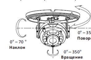
Рисунок 1-12 Настройка угла наблюдения камеры
