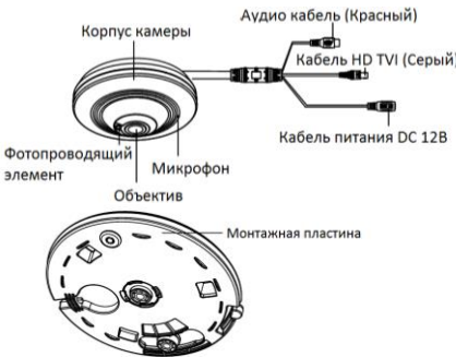
Рисунок 1-28 Панорамная камера
