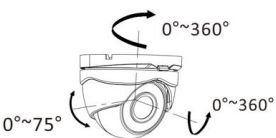
Рисунок 1-21 Настройка угла наблюдения камеры
