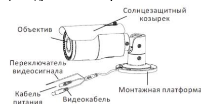
Рисунок 1-7 Цилиндрическая камера VI типа
