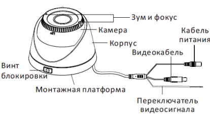
Рисунок 1-22 Камера «шар» VI типа
