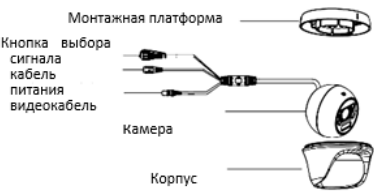
Рисунок 1-19 Камера «шар» IV типа
