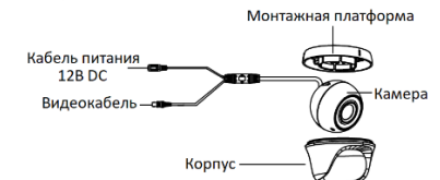
Рисунок 1-15 Камера «шар» I типа Поворот [0° — 360°]
