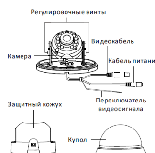
Рисунок 1-11 Купольная камера I типа
