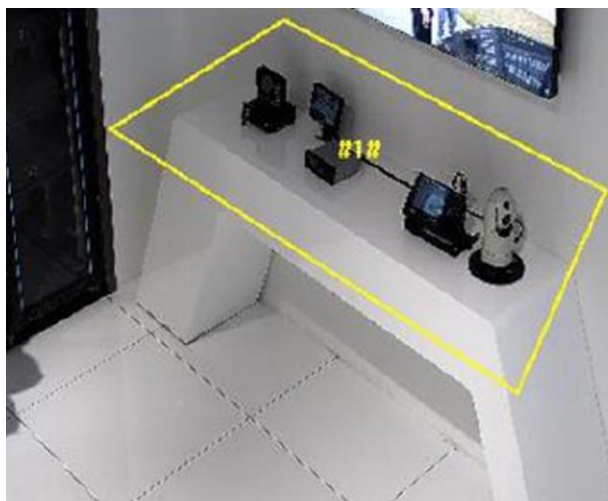
Рисунок 6-9 Настройка правил
