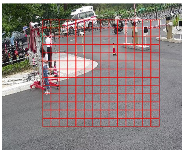
Рисунок 6-2 Настройка правил
