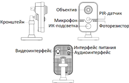
Рисунок 1-26 Компактная камера
