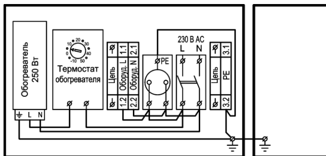
Рисунок 2 – Схема электрическая принципиальная
