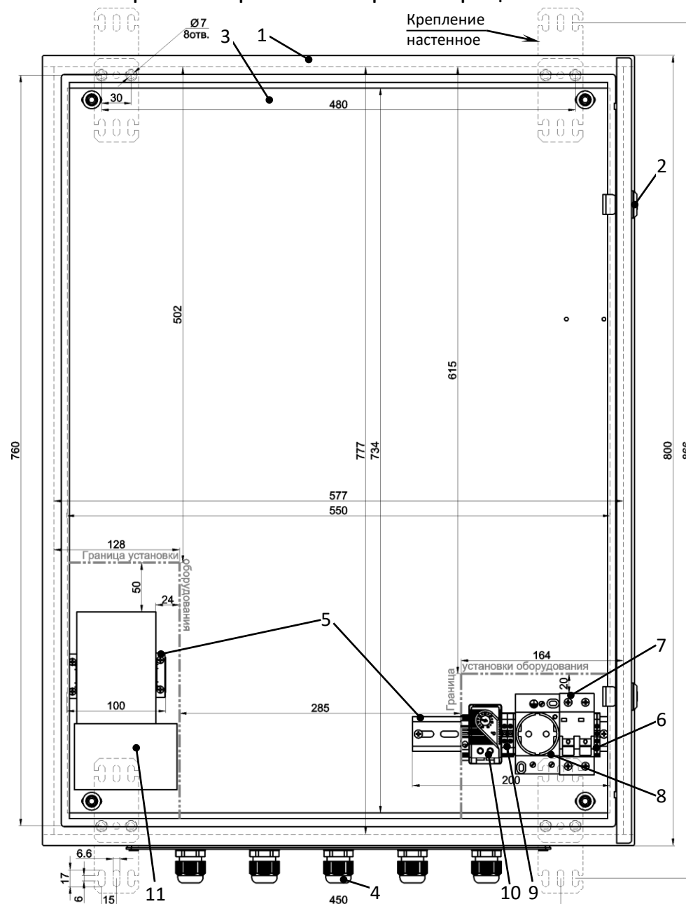
Рисунок 1 – Устройство шкафа
