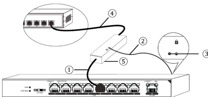
Рисунок 3.2 Подключение молниеотвода
