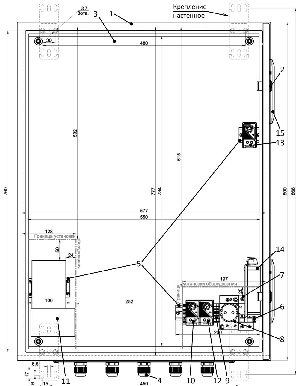
Рисунок 1 – Устройство шкафа
